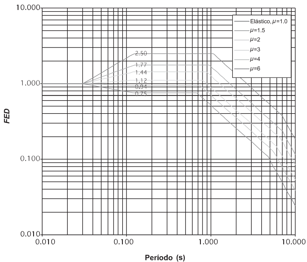
FIGURA 5.12. Factor espectral dinámico, FED , para sitios de cimentación tipo S_4 en zona sísmica IV (amortiguamiento z = 5\% ; ductilidades m = 1, 1.5, 2, 3, 4, 6 ).
