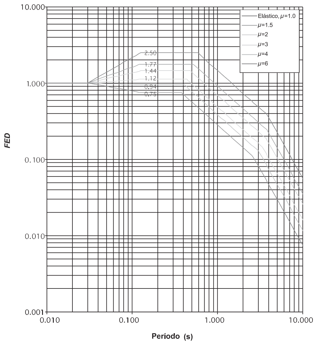
FIGURA 5.11. Factor espectral dinámico, FED , para sitios de cimentación tipo S_3 en zona sísmica IV (amortiguamiento \alpha = 5\% ; ductilidades m = 1, 1.5, 2, 3, 4, 6 ).
