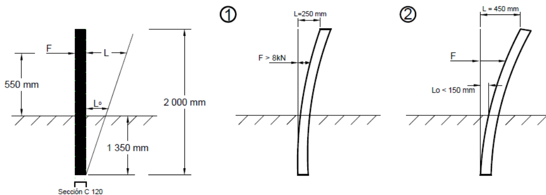
Figura 617-01 Ensayo estático in situ
